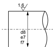
相配轴 Mating Shaft
